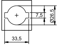
BAĞLANTI YUVASI
